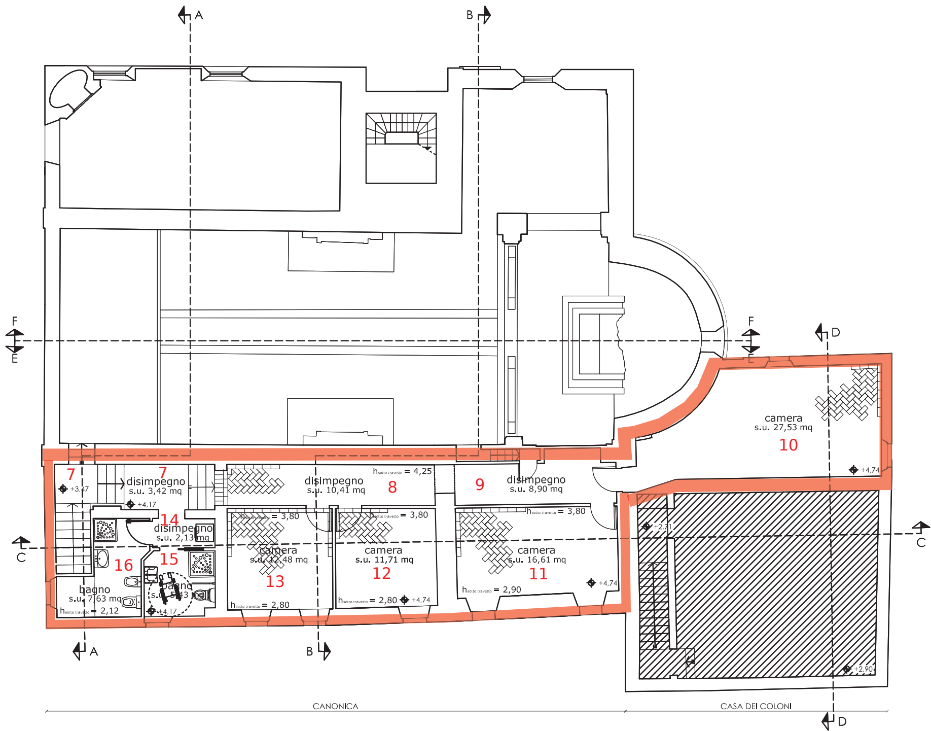
PIANTA PIANO PRIMO "CANONICA" scala 1:100
