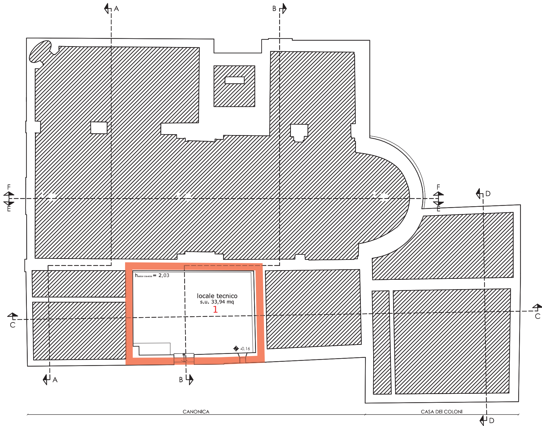
PIANTA PIANO SEMINTERRATO scala 1:100
