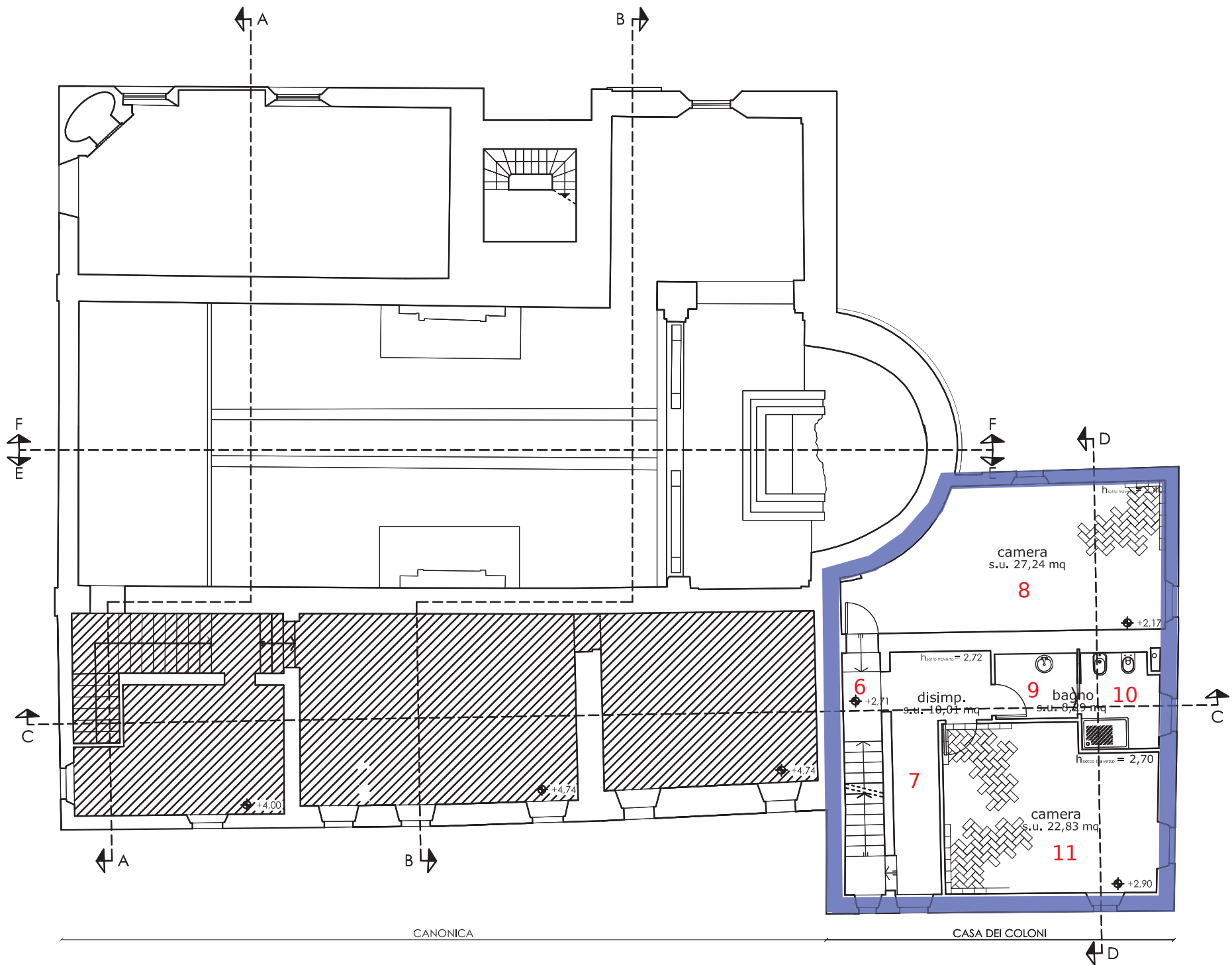
PIANTA PIANO PRIMO "CASA DEI COLONI" scala 1:100
